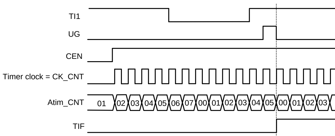
图26-41复位模式下的时序
