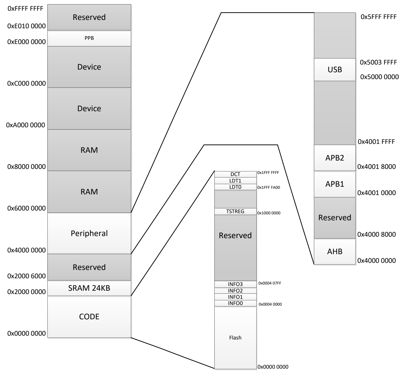
图 7-2FM33LC04x 总线地址
