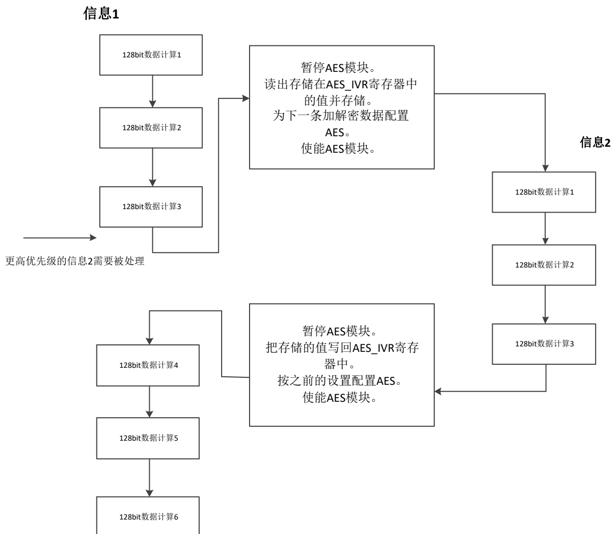
图 14-5 暂停模式流程
