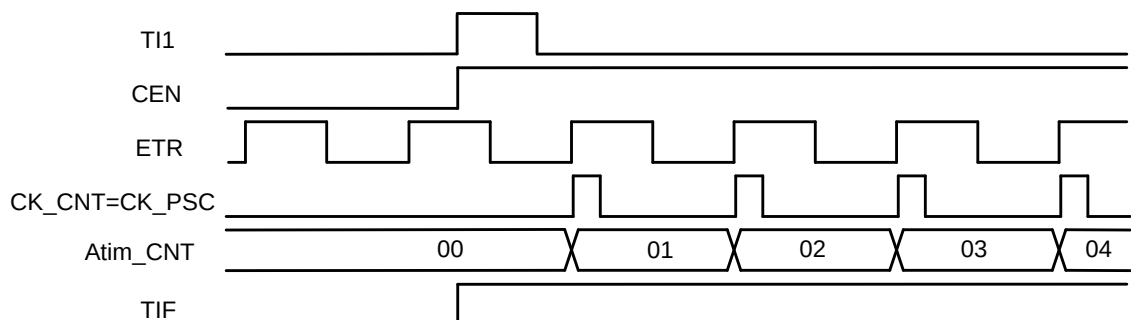
图26-44外部时钟模式2+触发模式下的时序
