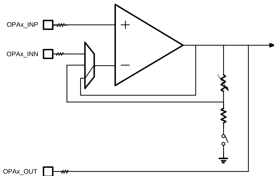
图 16-8OPA 缓冲器模式
