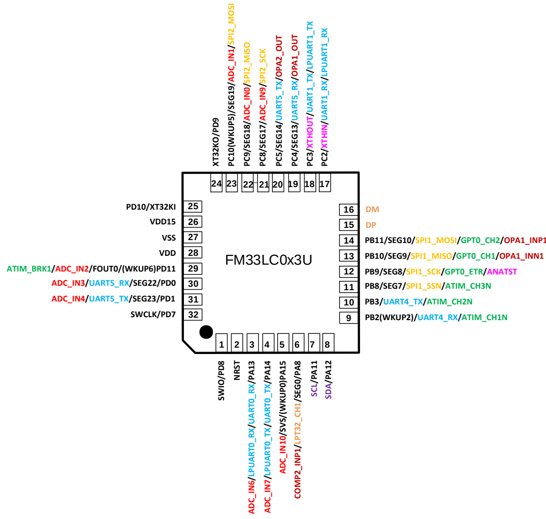
图 2-6FM33LC0x3U QFN32 封装图
