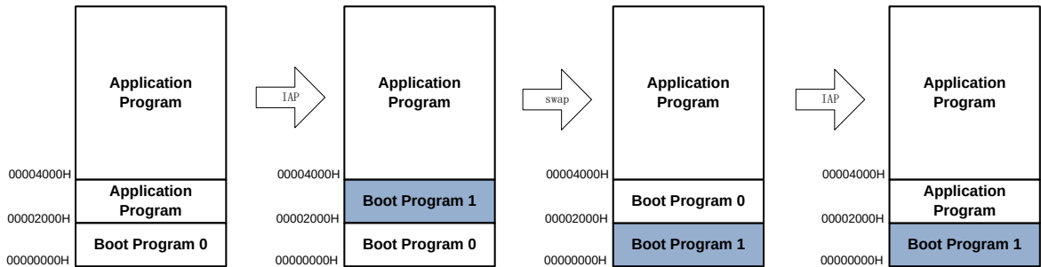
图 7-4Bootswap 示意图
