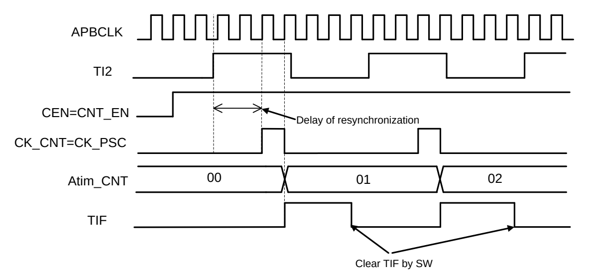
图 26-19 外部时钟模式 1 下的时序
