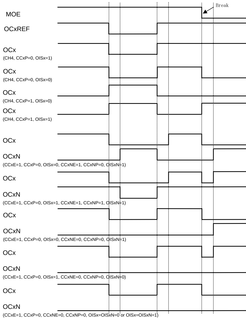
图26-36响应刹车的输出
