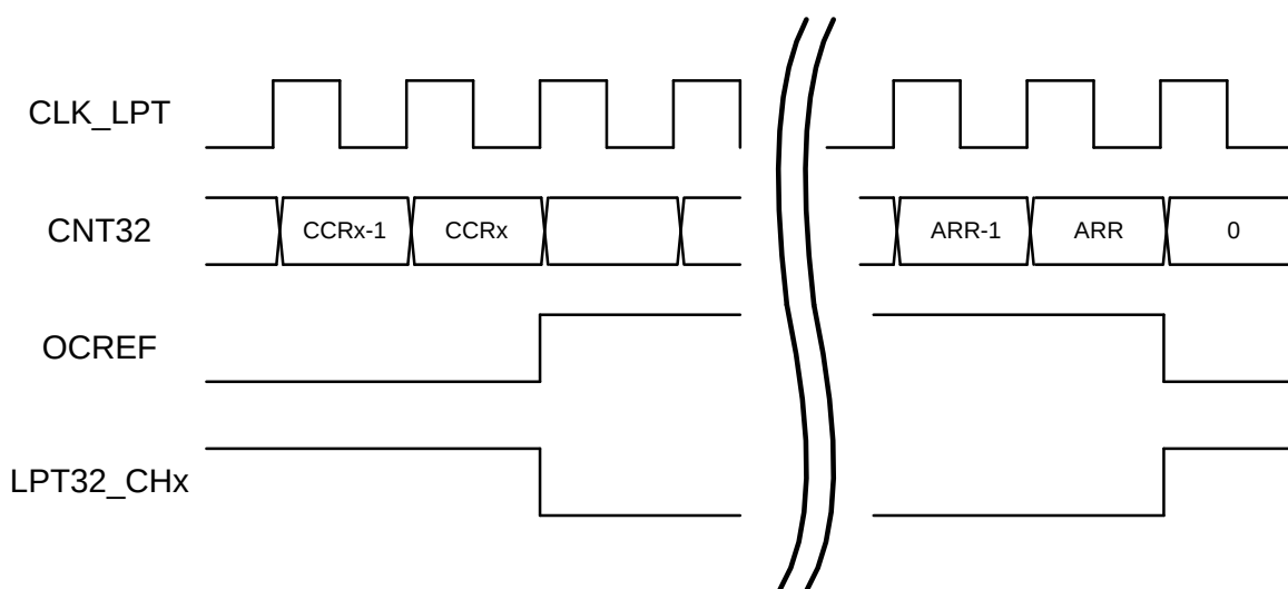
图 29-5 PWM 输出
